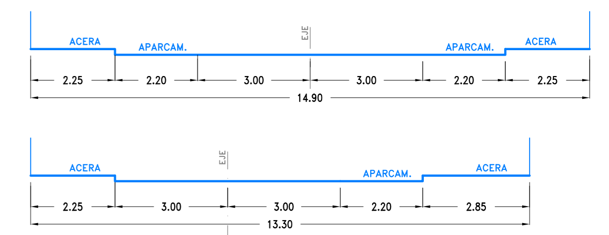
SECCIONES TIPO.- ESCALA 1/100
